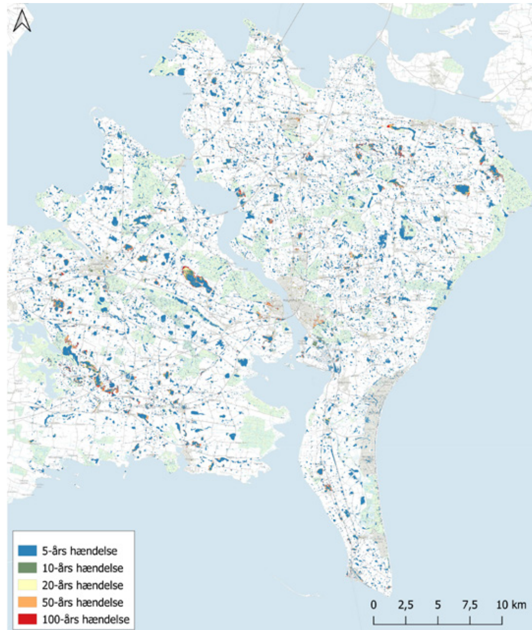
FIGUR 10.2: SANDSYNLIGHEDSSKORT OVER OVERSVØMMELSESOMRÅDER VED EN 5, 10, 20, 50 OG 100 ÅRS NEDBØRS-HÆNDELSE, FREMSKREVET TIL ÅR 2100 PBA. KLIMASCENARIET RCP8,5.
