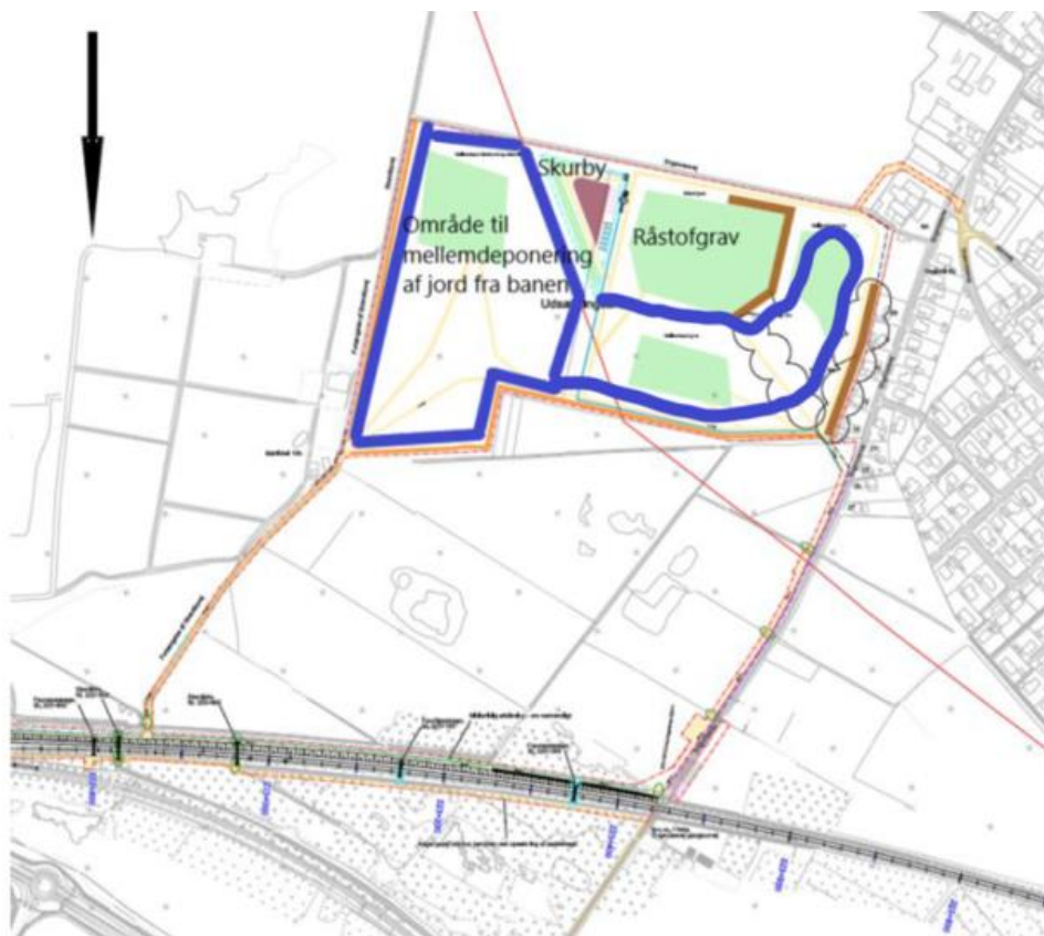
Figur 1: Indretning af byggeplads. § 19-pladsen anrettes inden for område markeret med blå. Bemærk, at nord vender ned.
