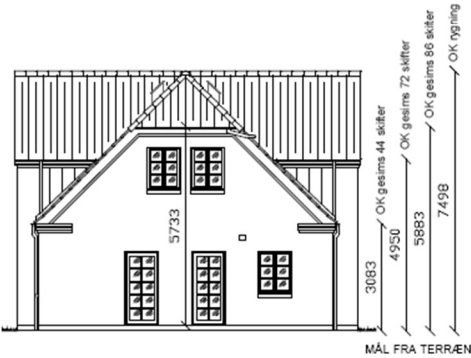
VEST GAVL
