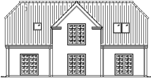
SYD FACADE
