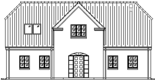
NORD FACADE
