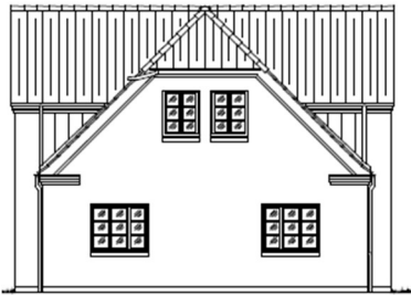
ØST GAVL
