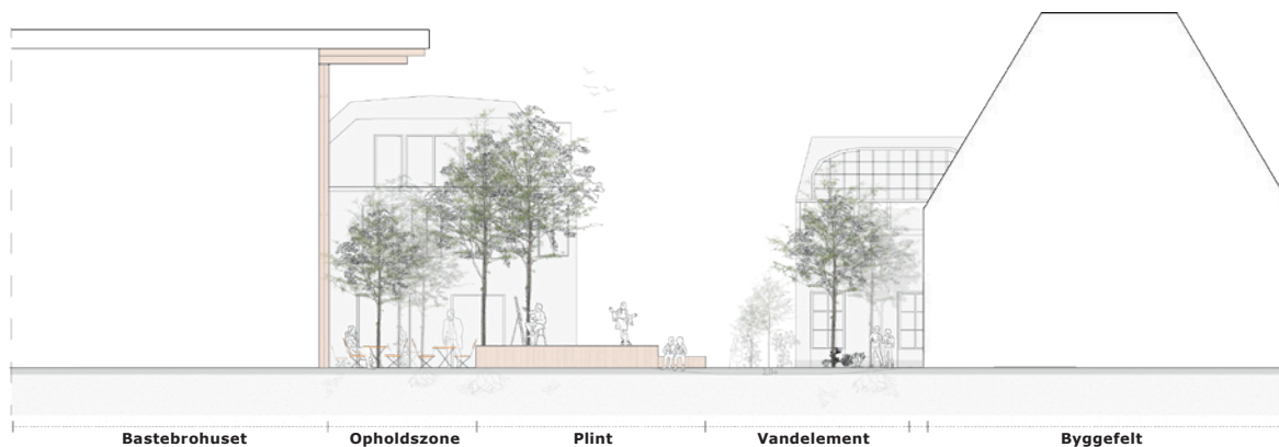
FIGUR 11. LÆNGDESNIET - SET FRA SUNDET OG IND I BROPLADSEN
