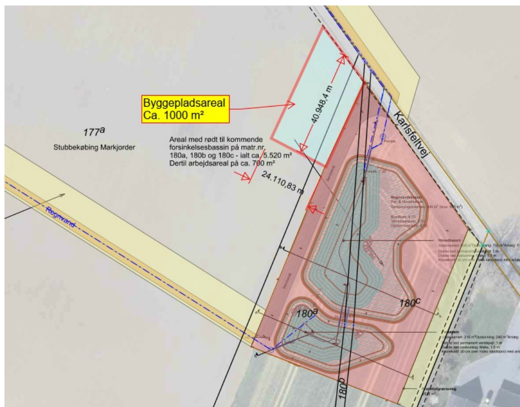
Luftfotoet viser placeringen af det ansøgte forsinkelsesbassin, samt den midlertidige byggeplads.
