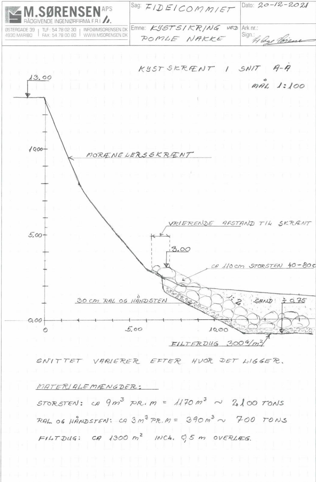
Snittegning udført af Rådgiver af det ansøgte kystbeskyttelses anlæg
