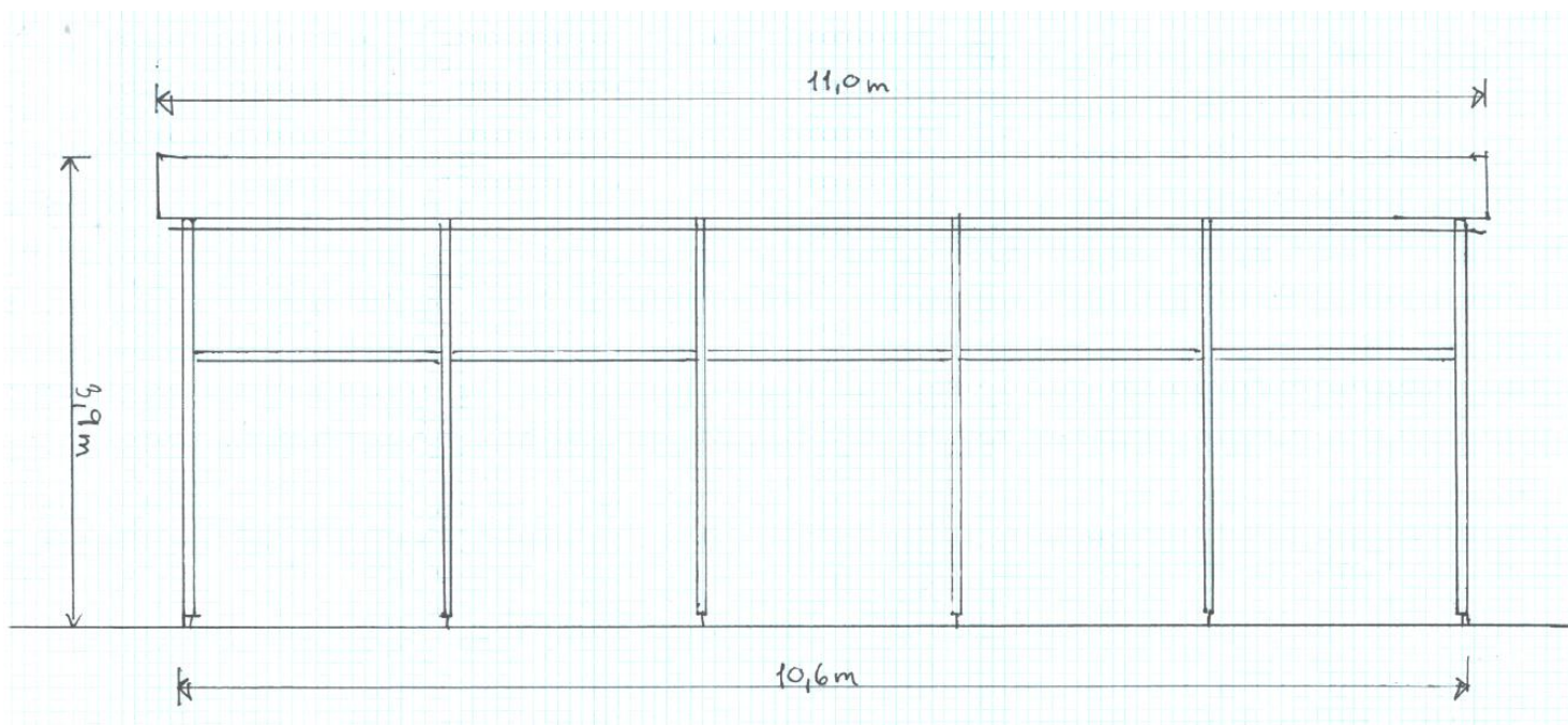
Tegning af nordsiden af facaden
