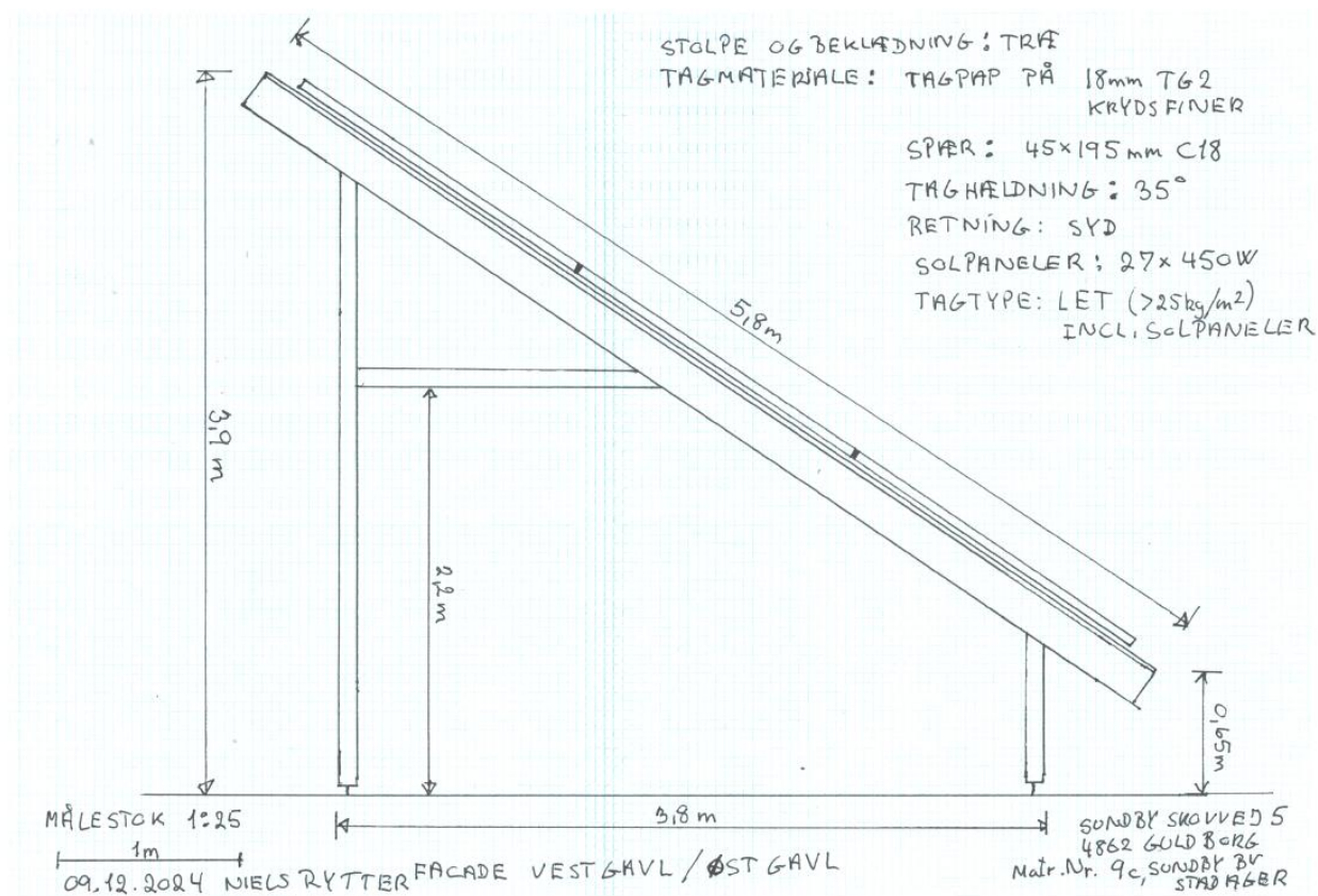
Snittegning af solcellerne
