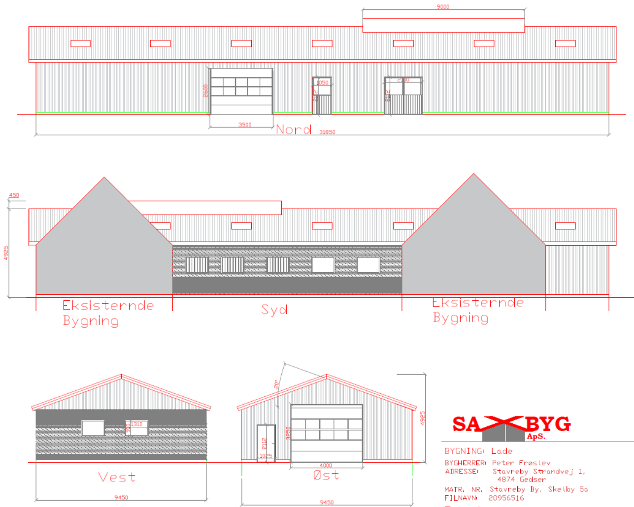
Tegninger af den ansøgte bygning
