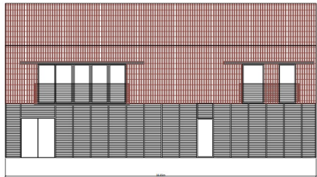
Opstalt 1:100 - Vest
